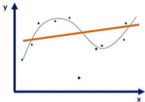
Subajuste
