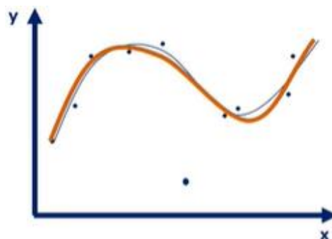
Ajuste Adequado
