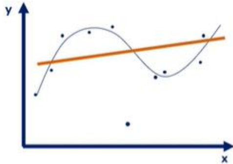
Subajuste
