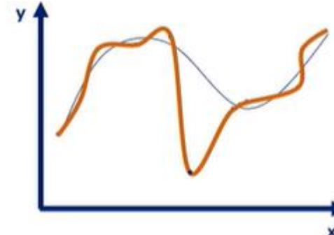
Sobrecaptação
