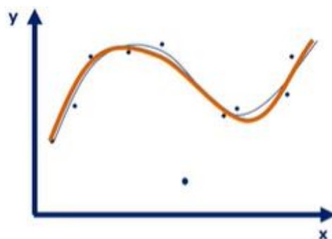
Ajuste Apropriado
