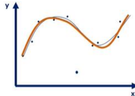
Ajuste Adequado
