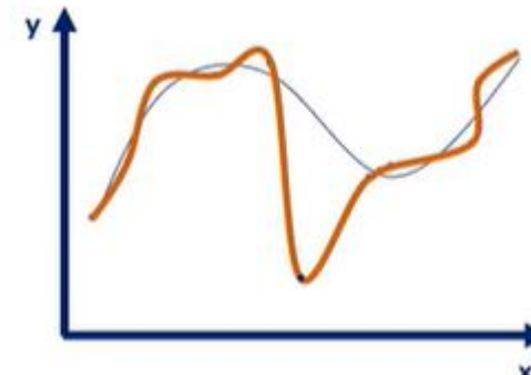
Sobreajuste
